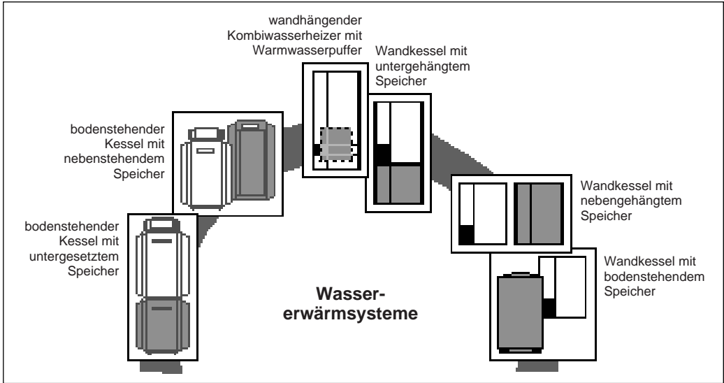
Varianten von Wassererwärmungssystemen, mit wandhängenden und bodenstehenden Kesseln und Speichern unterschiedlicher Art, jedoch im Design aufeinander abgestimmt (Bilder: Buderus Heiztechnik)
